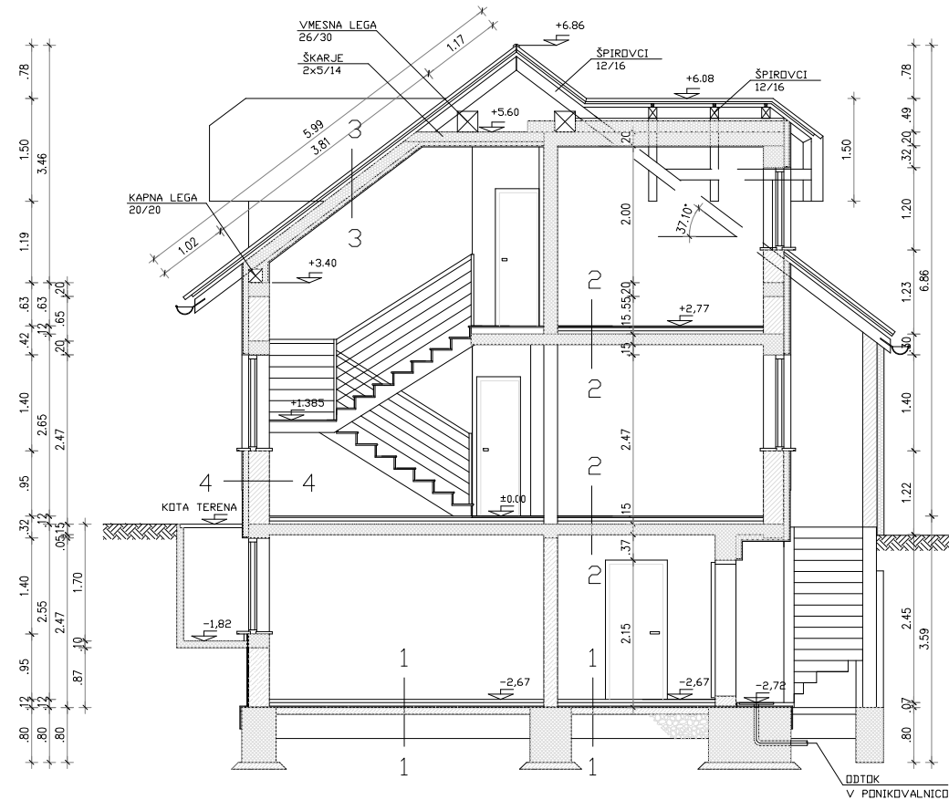
PREREZ B-B
